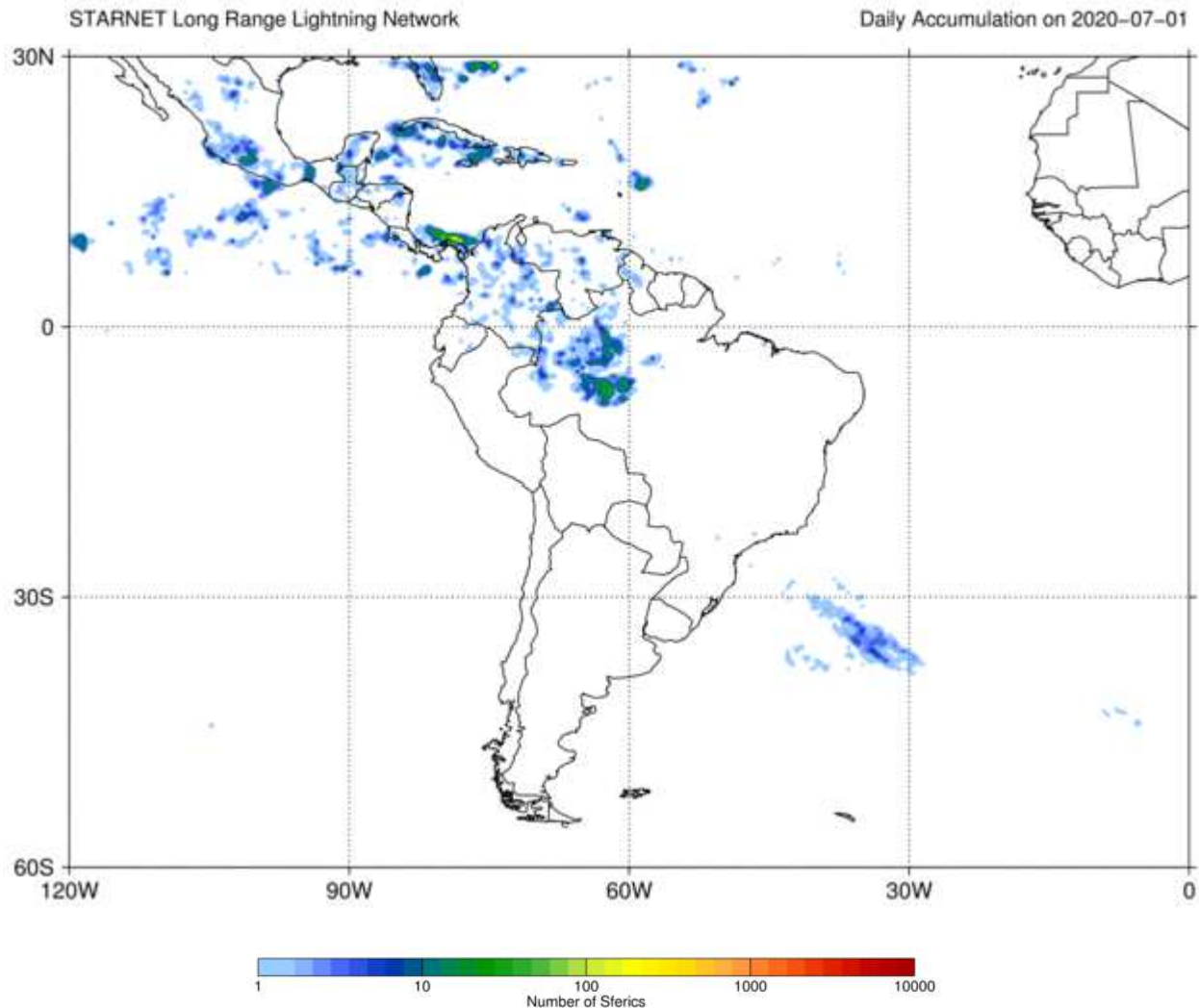
Figura 4 – Descarga elétrica acumulada: dia 01/07/2020 Fonte: Starnet-IAG-USP.
