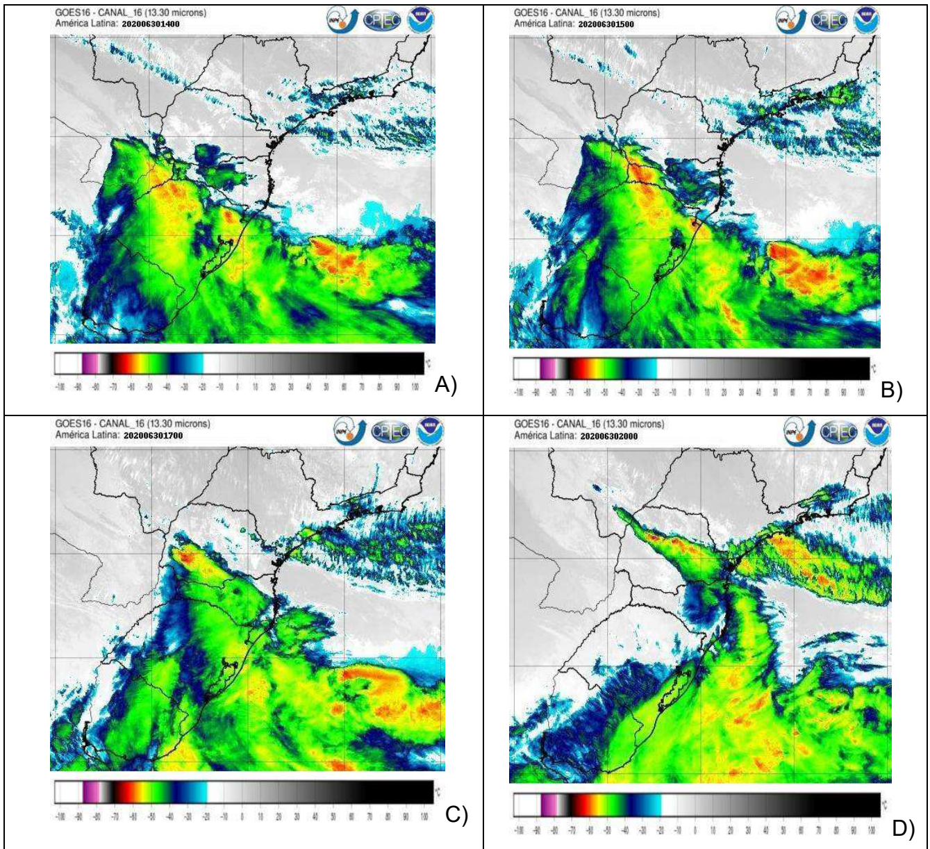
Figura 1 – Imagens realçadas do satélite GOES-16 do dias 30 de junho de 2020, horário local: A) dia 30 às 11:00h; B) dia 30 às 12:00h ; C) dia 30 às 14:00h e D) dia 30 às 17:00h. Fonte: CPTEC/INPE.
