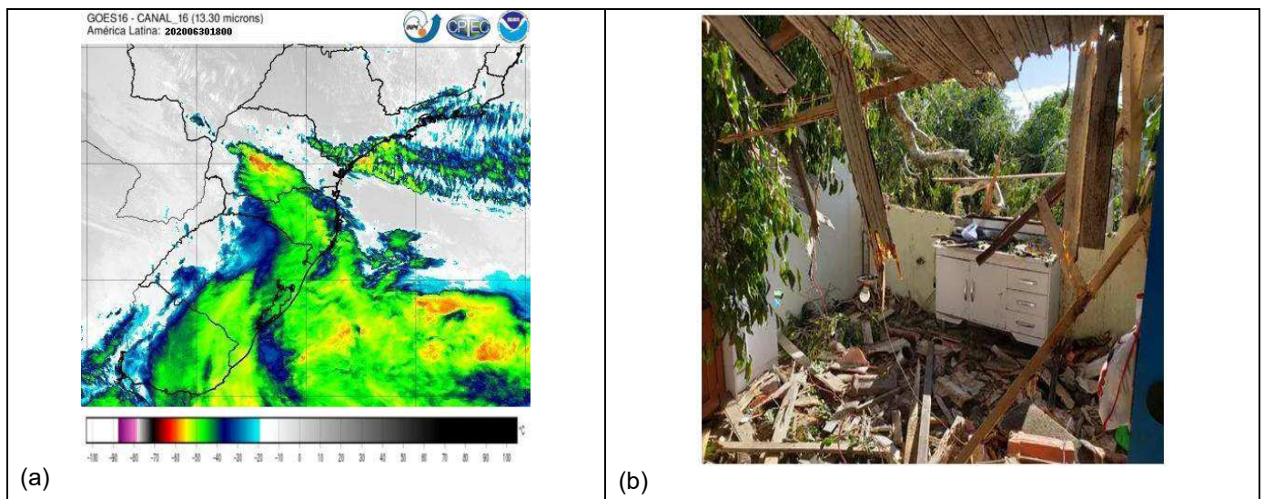
Figura 5 – (a) Imagem de satélite do Sul do Brasil no dia 30/06/2020, às 15h00min (horário local) (Fonte: CPTEC/INPE); (b) imagem de uma casa destruída no bairro de Ratores Florianópolis, devido a rajadas de vento (Fonte: NSCTOTAL).
