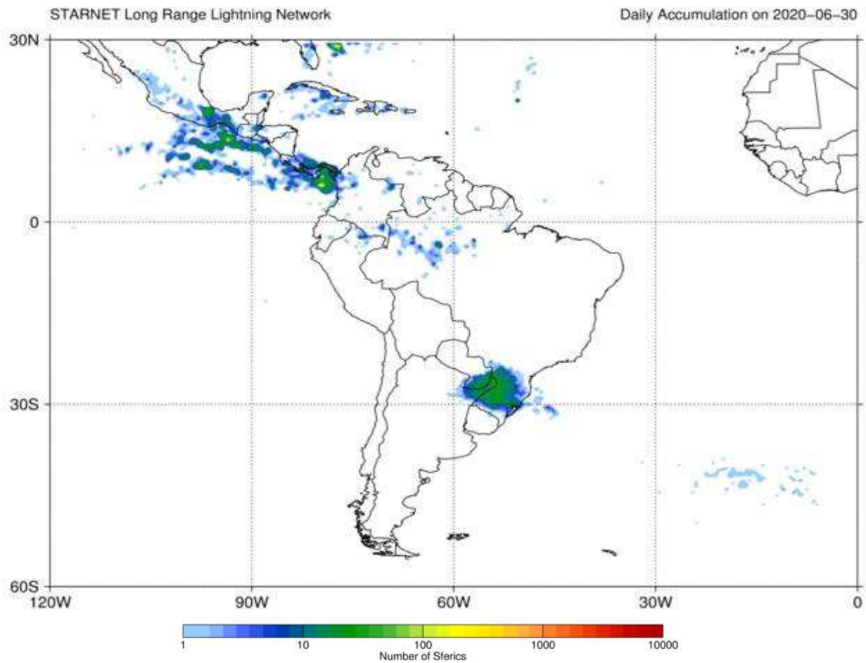
Figura 3 – Descarga elétrica acumulada: dia 30/06/2020 Fonte: Starnet-IAG-USP.
